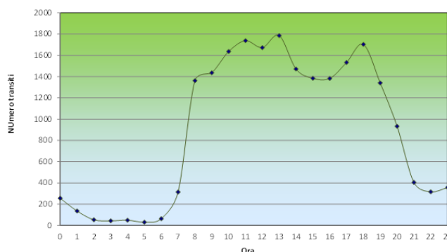
FLUSSI VEICOLARI "LITORANEA PORTO" - DAL 26/01/2021 AL 04/03/2021 Giorno Tipo Transiti in uscita Mezzi Leggeri
